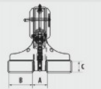
Einfahrtaschen-Innenmaße (mm)
